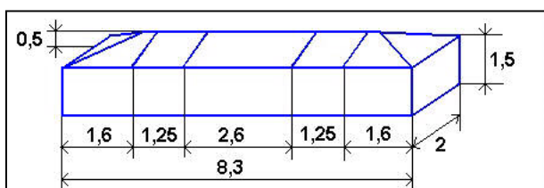
Obr.1 – Námězník-nákres
