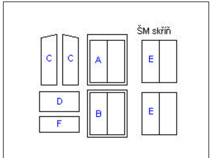
Obr. 8 - Střihy ŠM skříně 1:1 pro H0
